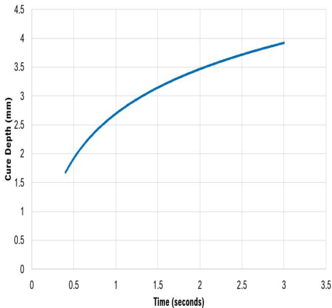
BlueWave® MX-150 PrimeCure® 385 nm (15 W/cm 2 )
